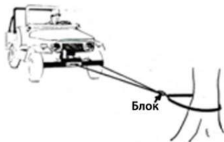
Рис. 20.4 Использование блока даёт механическое усилие 2:1. К тому же вдвое уменьшается нагрузка на трос и лебёдку. Соответственно, мотор будет крутить быстрее и с
