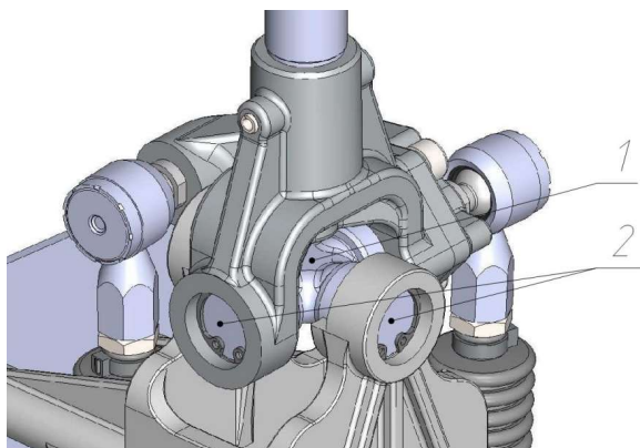
Рис. 6.5 Шарнирный узел мастер-опоры 1 – крестовина; 2 – игольчатый подшипник.
