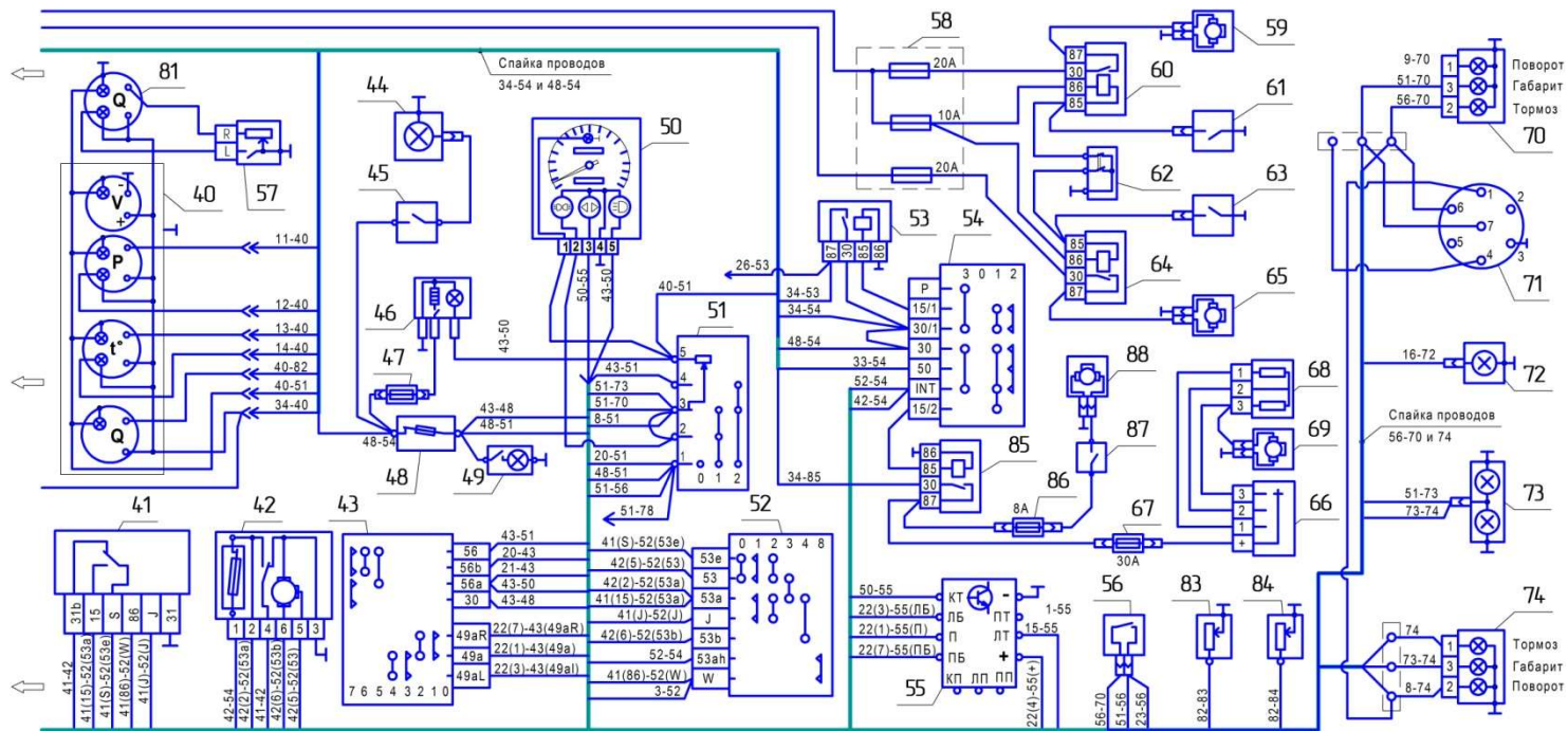
Рис. 6.22 (часть 2) Базовая электрическая схема ВТС
