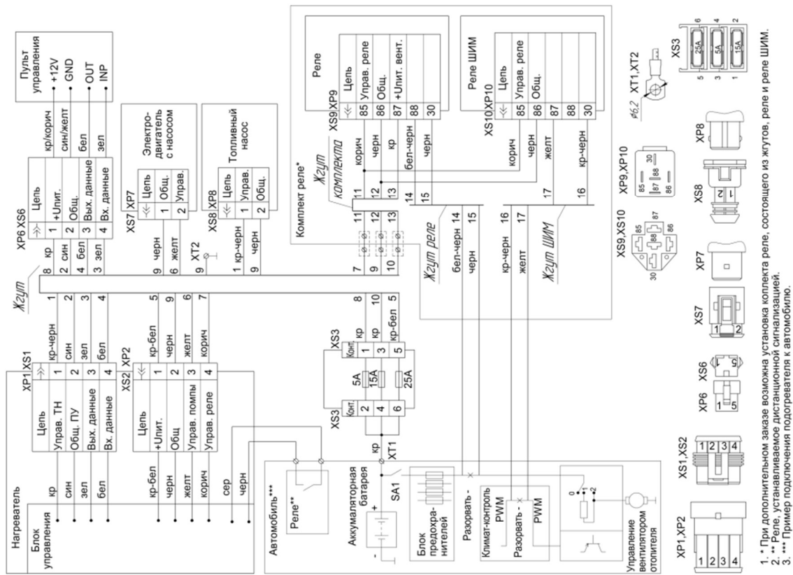
Рис. 20.12 Электрическая схема подключения подогревателя
