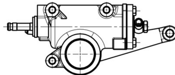
Рис. 6.17. Установка рулевой сошки
