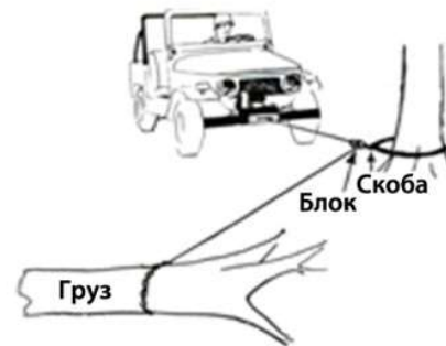
Рис. 20.6 Пример того, как с помощью блока можно менять направление тяги. Блок подсоединяется к древозащитной ленте с помощью соединительной скобы
