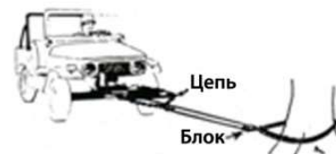
Рис. 20.5 В основном то же, что на рис. 20.4. Цепь с распределителем помогает равномерно распределить нагрузку по составным частям автомобиля.
