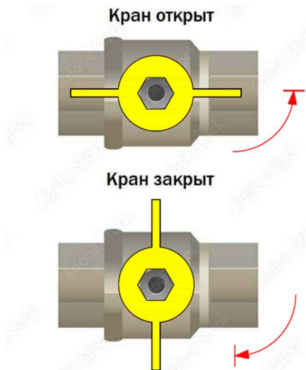
Рис. 20.2 Положения рукоятки колесного крана
