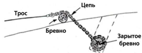
Рис. 20.10 Зарытое в землю бревно – отличный якорь. При необходимости вместо бревна можно использовать целый ряд предметов, например, металлическую балку, трубу или даже большую канистру.
