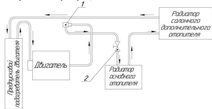
Рис. 6.35. Система отопления:
