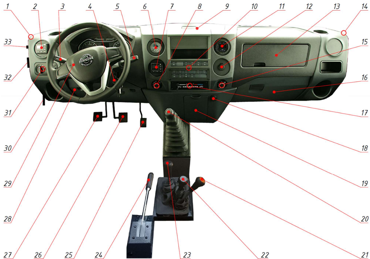
Рис. 5.4 Органы управления
