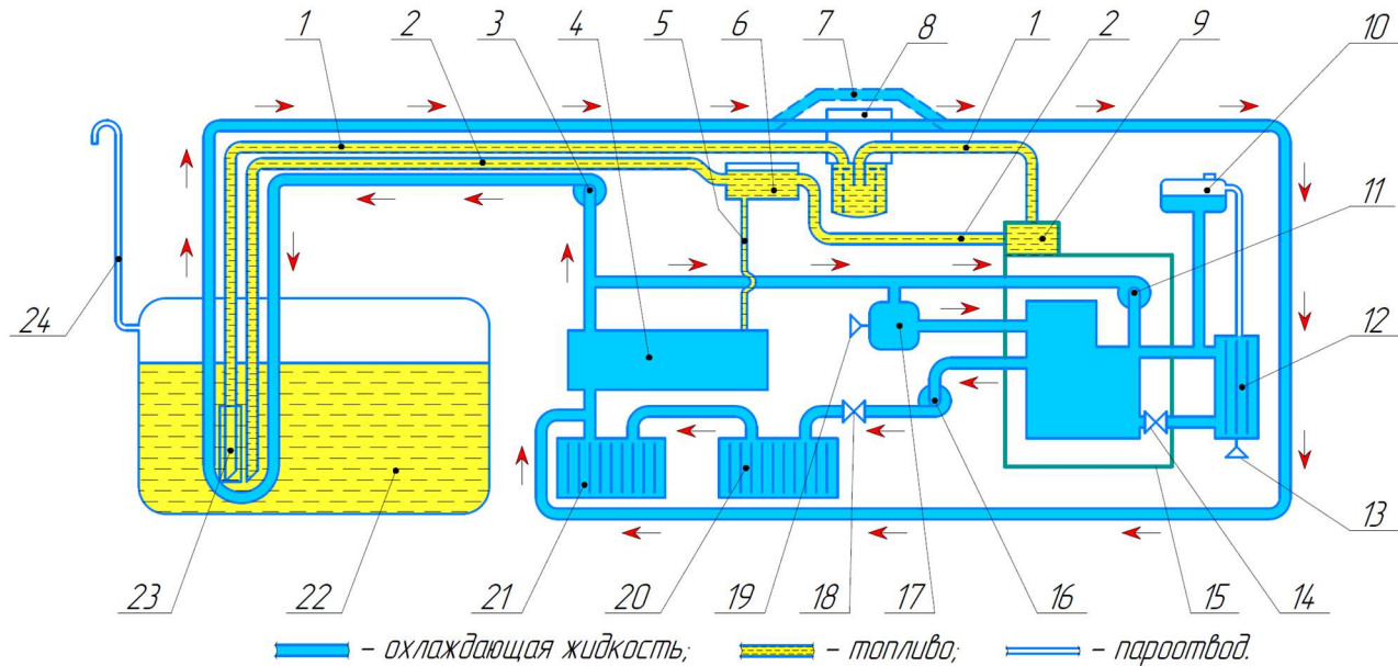
Рис. 20.19 Схема работы системы жидкостного подогрева топливной магистрали
