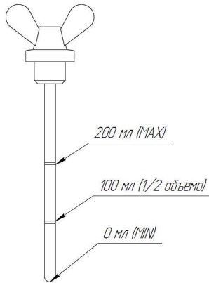
Рисунок 20.3. Указатель уровня антифриза
