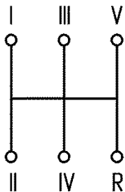
Рис. 6.1 Схема переключения коробок передач ГАЗ А63R43, Hyundai DYMOС и ГАЗ А31R32
